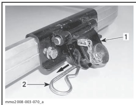
СЦЕПНОЕ УСТРОЙСТВО (ТИПА С) 1. Сцепное устройство 2. Проволоочный фиксатор
