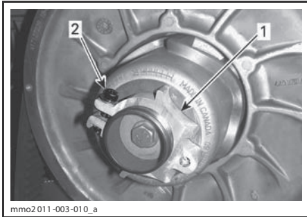
mm02011-003-010_a 1. Регулировочная муфта 2. Фиксирующий винт
