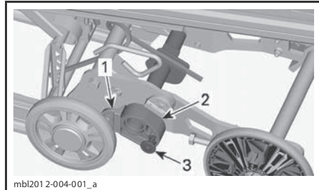
РЕГУЛЯТОР КУЛАЧКОВОГО ТИПА — АМОРТИЗАТОР MOTION CONTROL
