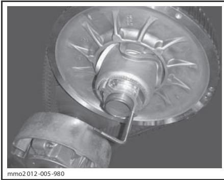
mm02012-005-980 ПРИСПОСОБЛЕНИЕ ДЛЯ РАЗВЕДЕНИЯ ШКИВА ВСТАВЛЕНО В РЕГУЛИРОВОЧНУЮ МУФТУ
