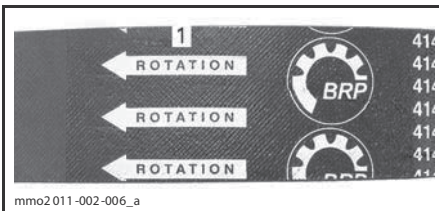
mm02011-002-006_a 1. Стрелки, указывающие направления рабочего движения ремня
