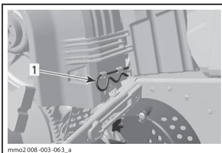
1. Проволочный фиксатор
