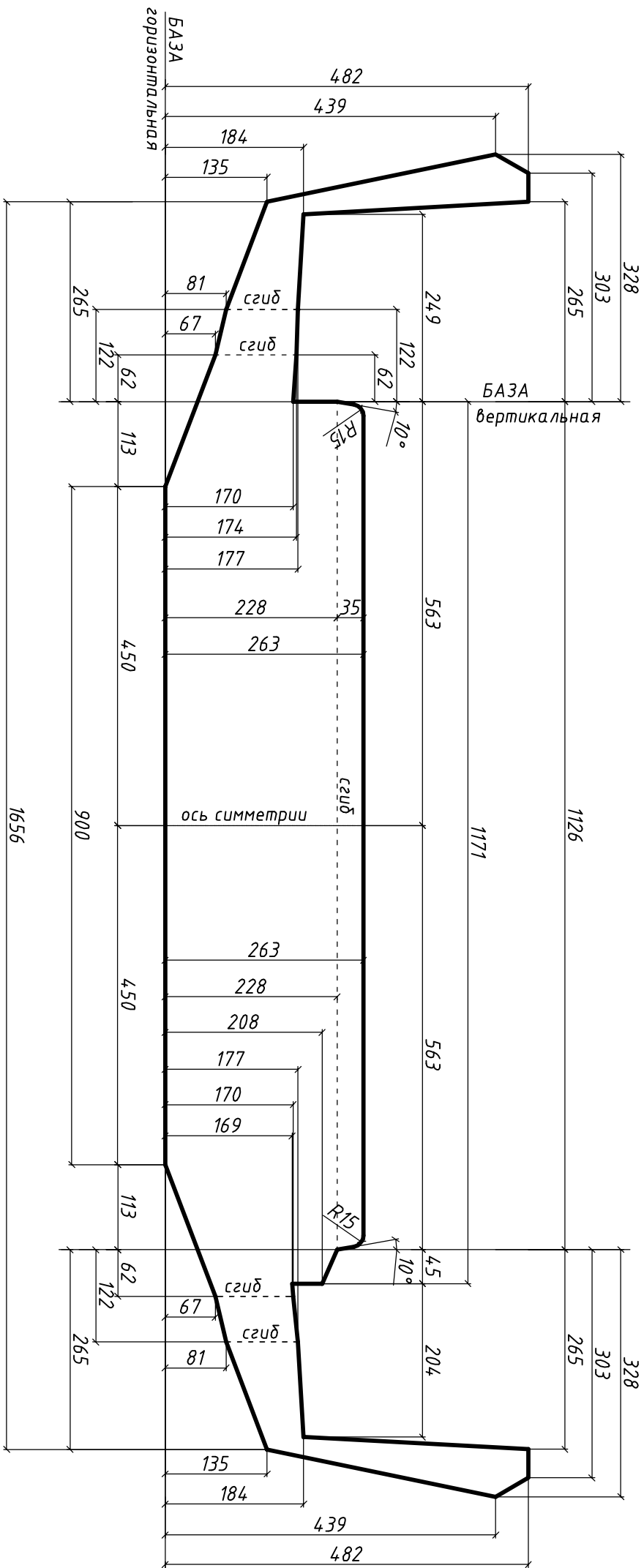
Развертка детали 1 (верхняя часть багнера) Черт. 1 – разметка листа (сталь 3 мм)
