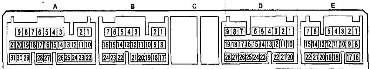
Выходы электронного блока управления (2ZZ-GE).
