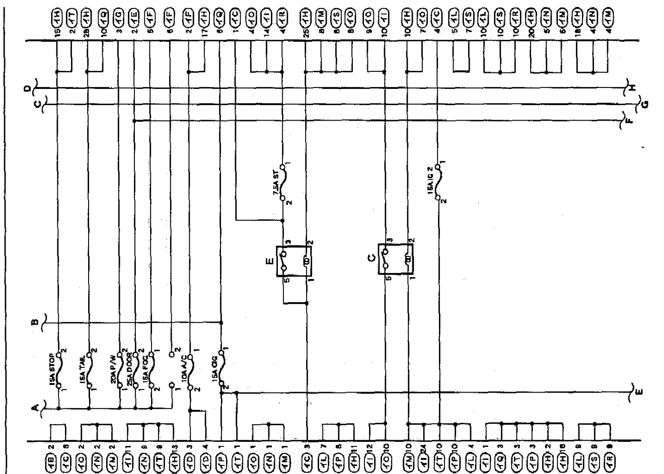
Монтажный блок под панелью приборов (внутренние цепи).
