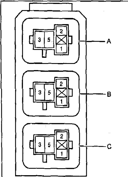
Блок реле дополнительного оборудования.
