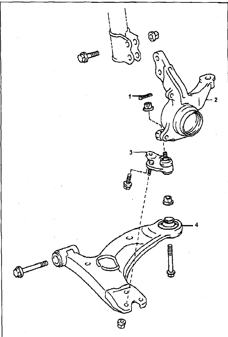
Нижний рычаг передней подвески. 1 - шплинт, 2 - поворотный кулак, 3 - нижняя шаровая опора, 4 - нижний рычаг передней подвески.
