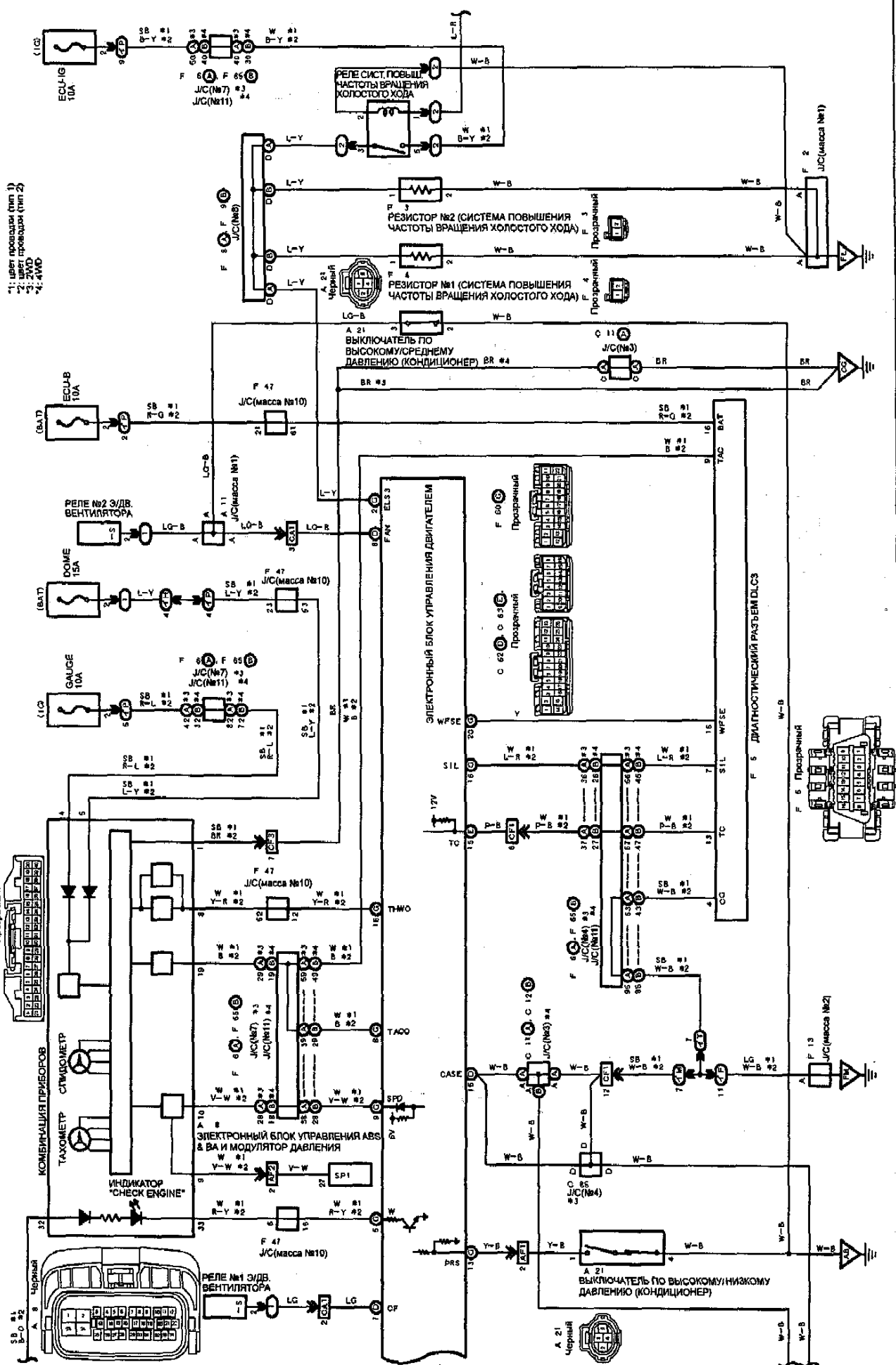
Схема 4 (продолжение).
