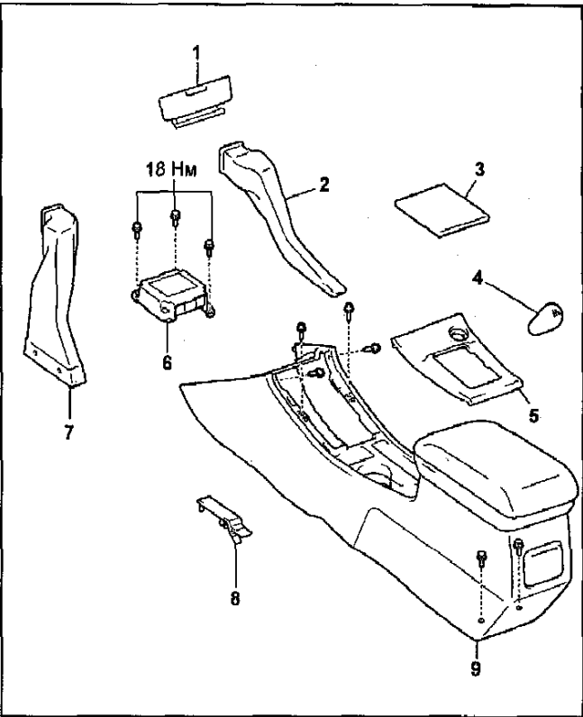
Снятие и установка блока управления SRS. 1 - пепельница, 2 - задний воздуховод №2, 3 - коврик ящика центральной консоли, 4 - ручка рычага выбора передач (МКПП), 5 - накладка центральной консоли, 6 - блок управления SRS, 7 - задний воздуховод №1, 8 - заглушка отверстия рычага стояночного тормоза, 9 - веще- вой ящик центральной консоли.
