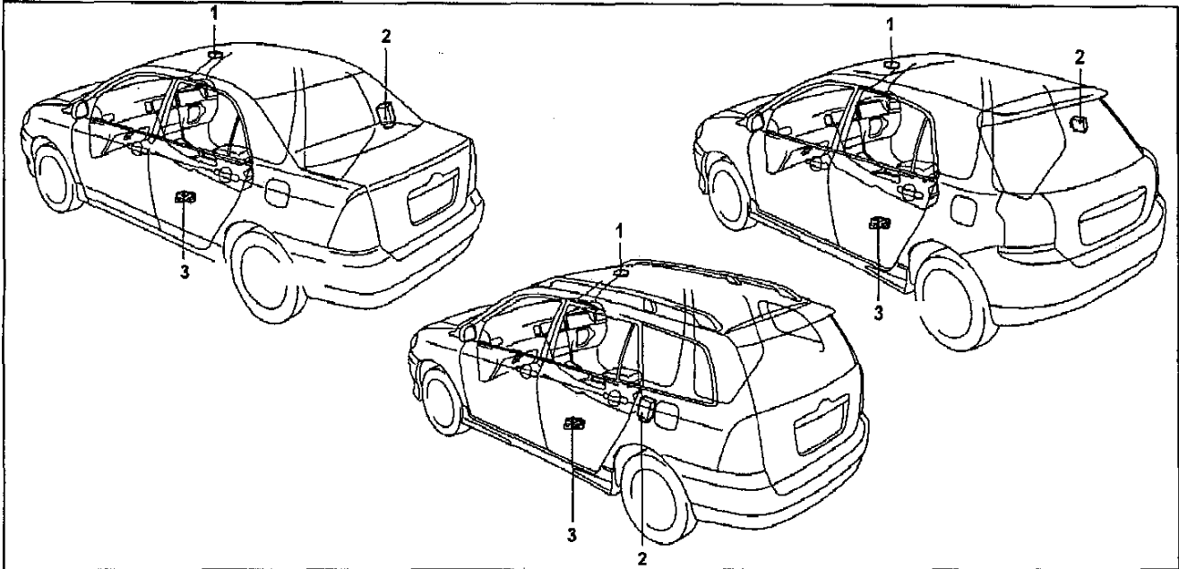
Расположение компонентов на кузове. 1 - лампа местной подсветки, реле и переключатель управления люком, 2 - блок управления центральным замком, 3 - датчик замедления (модели 4WD), датчик замедления и датчик крена (модели с VSC).
