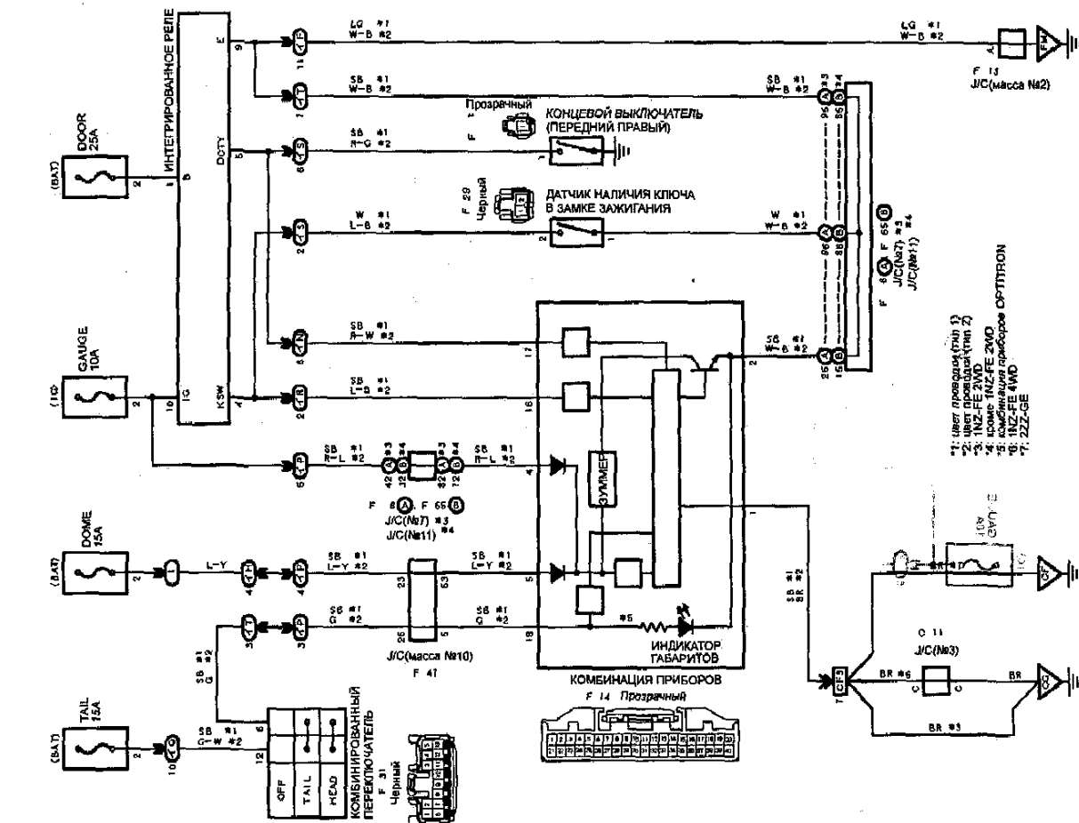
СИСТЕМА ПРЕДУПРЕЖДЕНИЯ ОБ ОСТАВЛЕННОМ В ЗАМКЕ ЗАЖИГАНИЯ КЛЮЧЕ (ХЭТЧБЕК)
