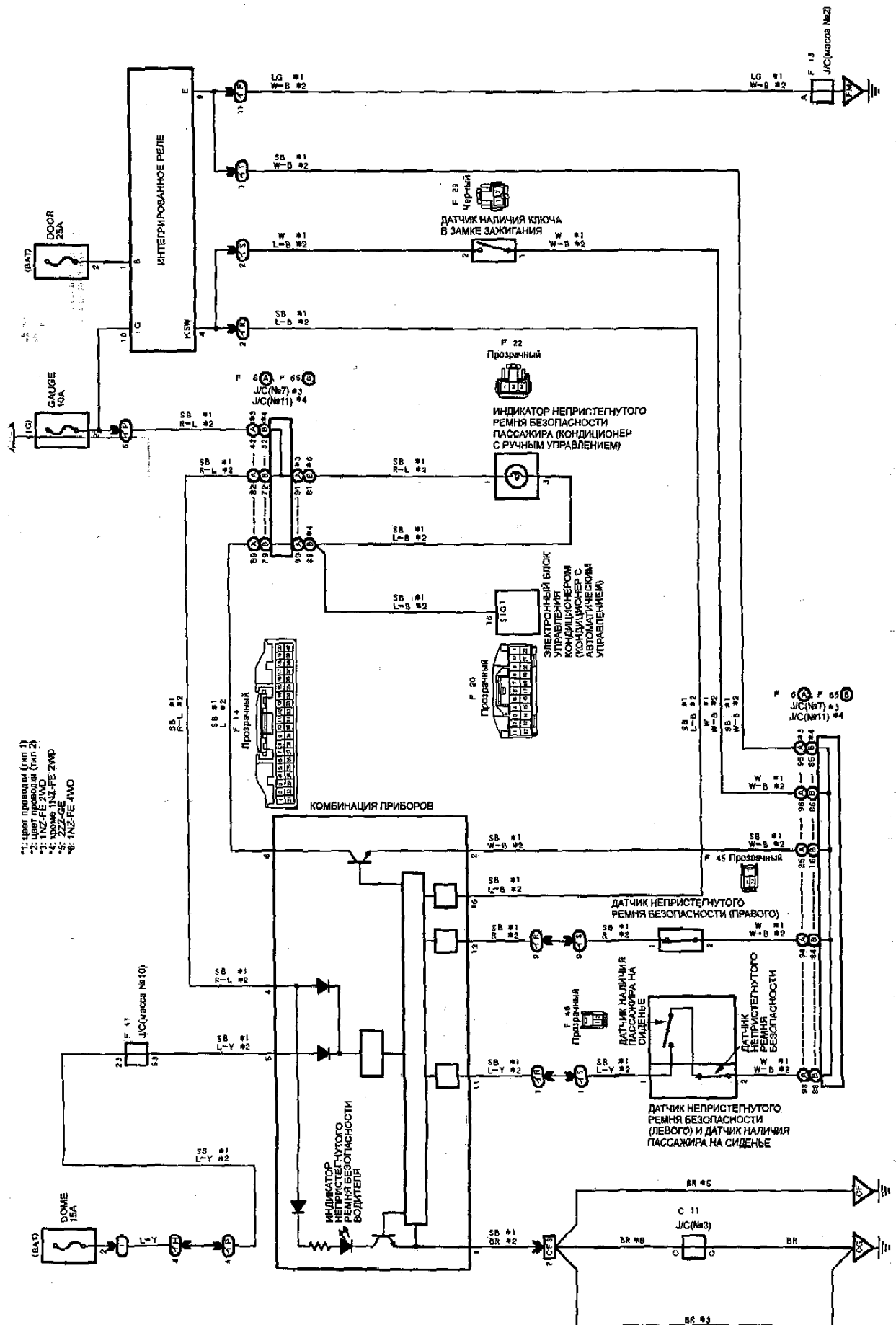
СИСТЕМА ПРЕДУПРЕЖДЕНИЯ О НЕПРИСТЕГНУТОМ РЕМНЕ БЕЗОПАСНОСТИ (ХЭТЧБЕК)
