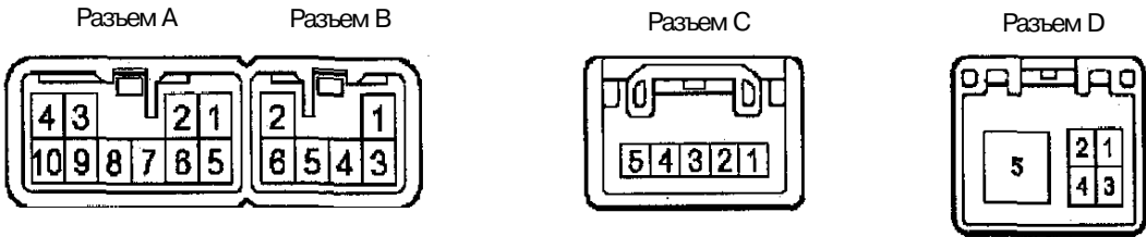
Разъем радиоресивера (блока MultiVision).
