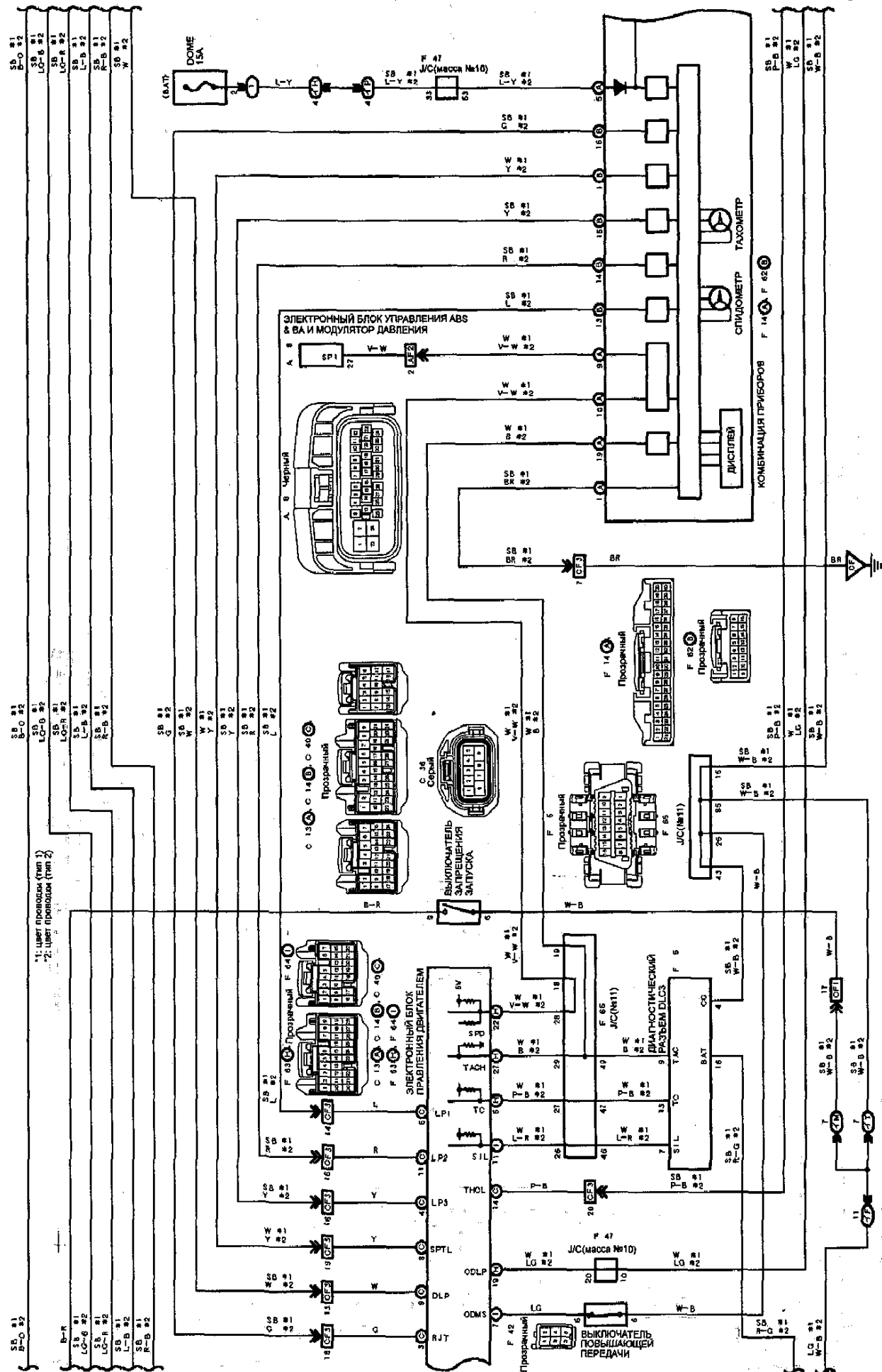
Схема 14 (продолжение).
