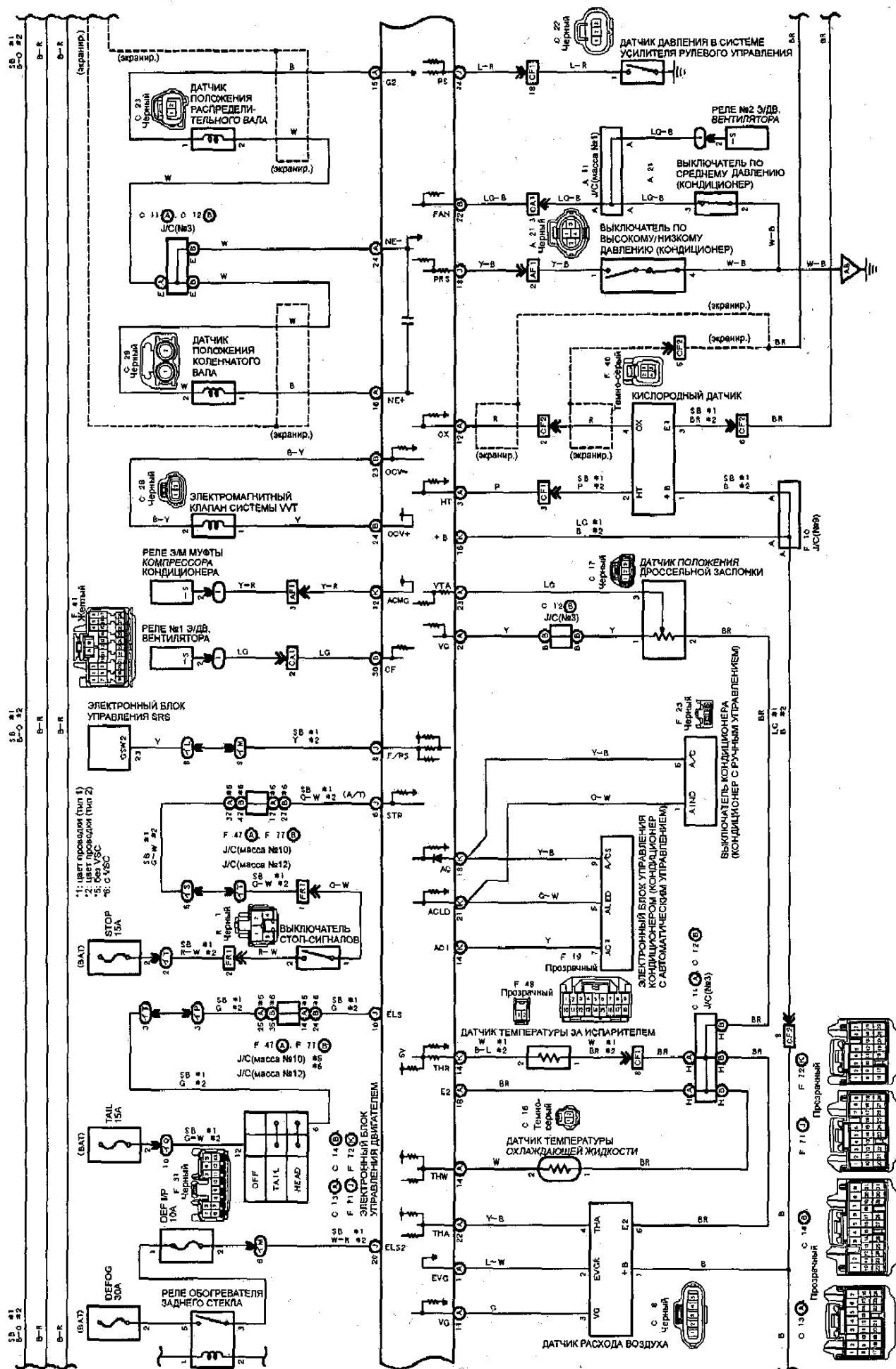
Схема 3 (продолжение).
