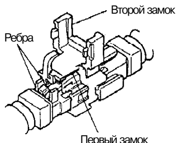
Первый замок открыт (второй закрыть нельзя)
