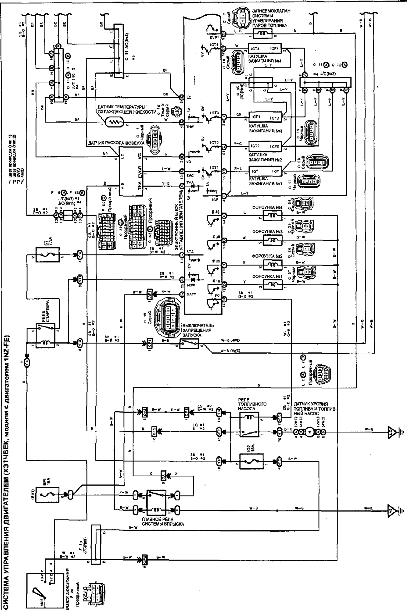
Схема 4.
