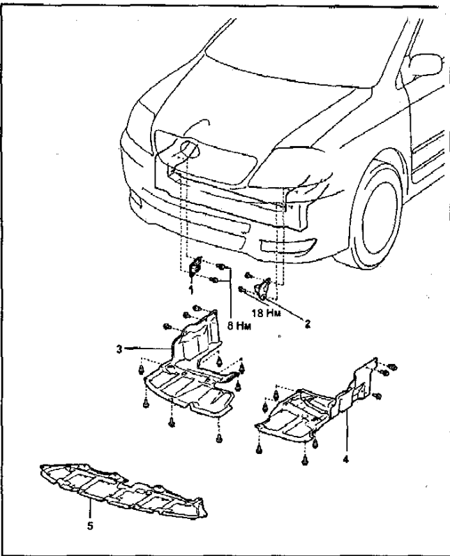
Снятие и установка передних боковых датчиков SRS. 1 - правый передний датчик SRS, 2 - левый передний датчик SRS, 3 - правый кожух защиты двигателя, 4 - левый кожух защиты двигателя, 5 - центральный кожух защиты двигателя.
