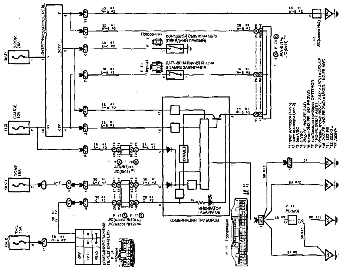
СИСТЕМА ПРЕДУПРЕЖДЕНИЯ ОБ ОСТАВЛЕННОМ В ЗАМКЕ ЗАЖИГАНИЯ КЛЮЧЕ (СЕДАН, УНИВЕРСАЛ)
