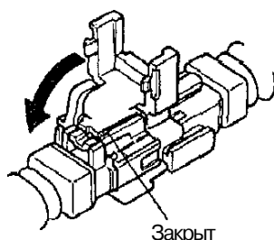
• Первый замок закрыт (разрешение закрытия второго замка)
