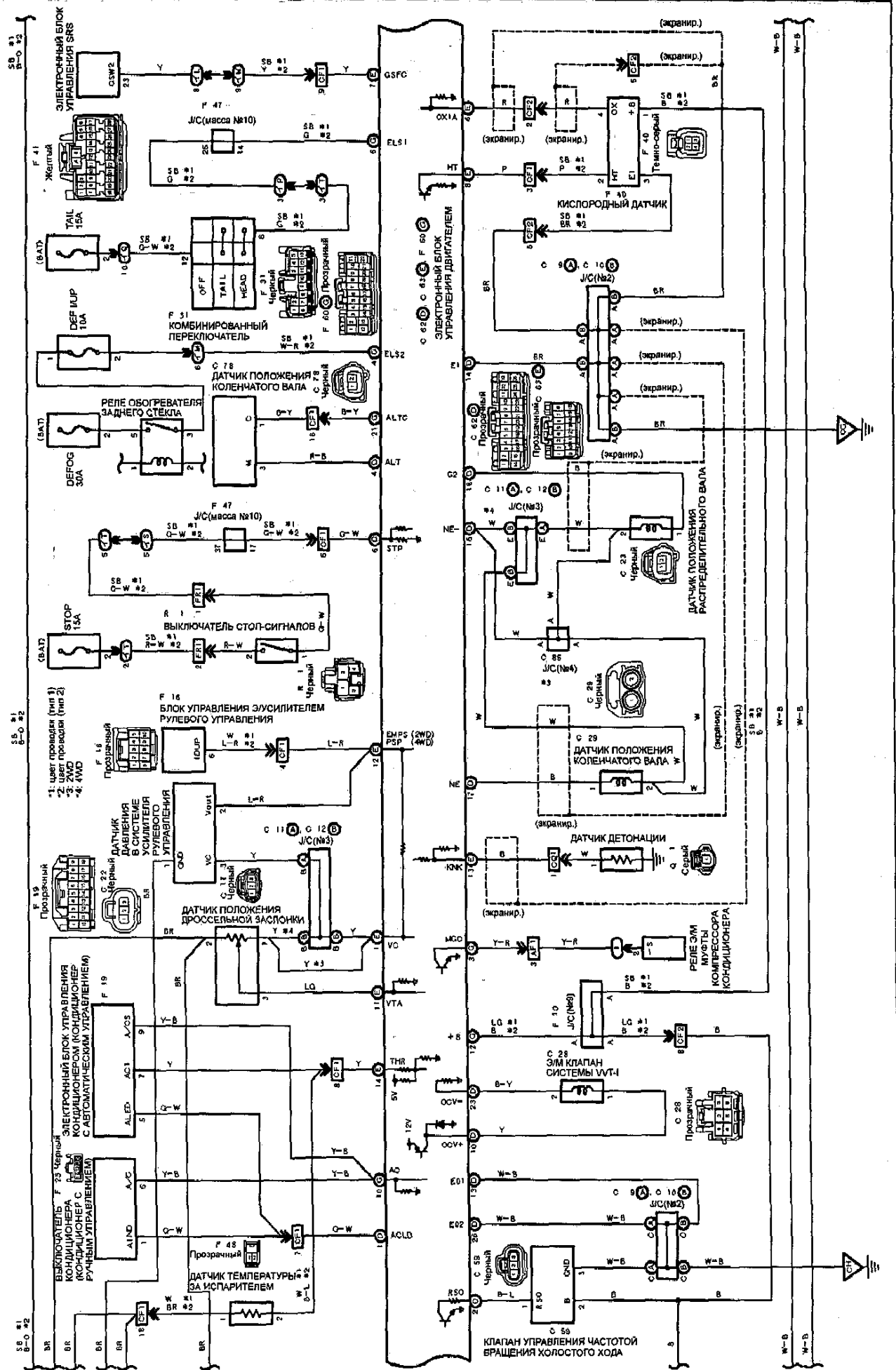
Схема 4 (продолжение).
